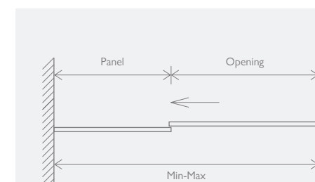
SLIDING DOOR
